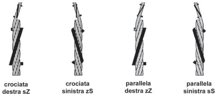
fig. 2 - senso di avvolgimento della fune
