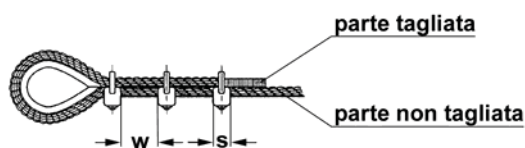
fig. 1 – posizionamento morsetti
