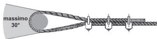
fig. 2 – angolo massimo dell'asola
